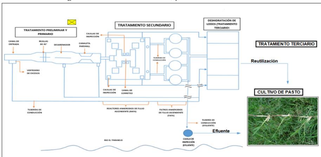
Figura 1. Esquema general de la PTAR del municipio de Timaná.
