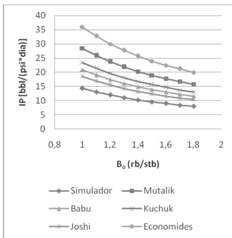
Figura 3. Comportamiento de la productividad del pozo variando el factor volumétrico del crudo.
