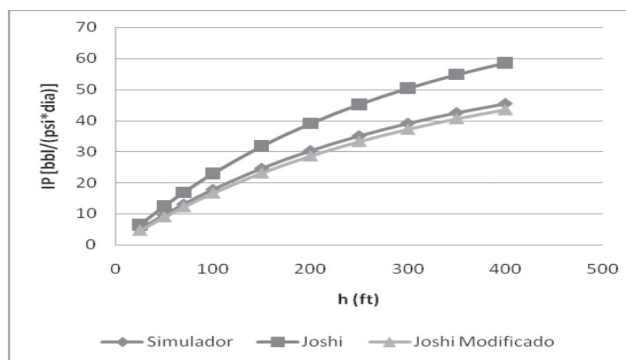
Figura. 12. Comportamiento de la productividad del pozo variando el espesor de la capa.
