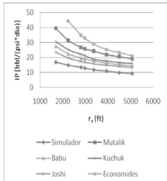
Figura 8. Comportamiento de la productividad del pozo variando el radio externo de frontera.
