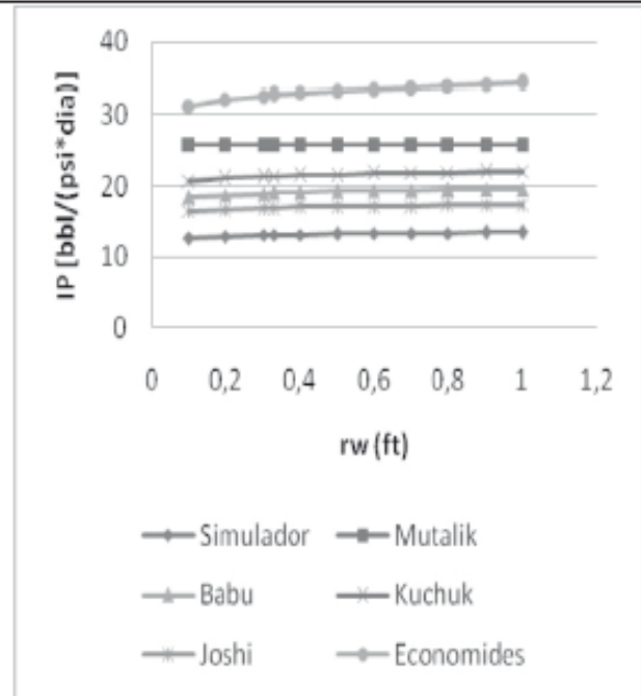
Figura 7. Comportamiento de la productividad del pozo variando el radio del pozo.
