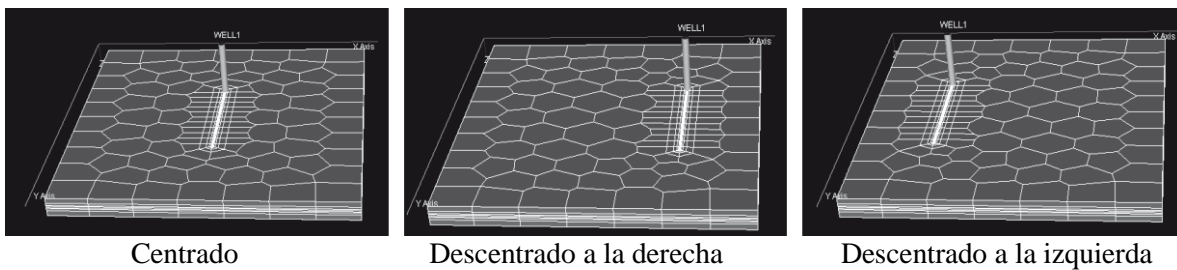
Figura 11. Esquemas de ubicación del pozo horizontal vistas en el simulador.
