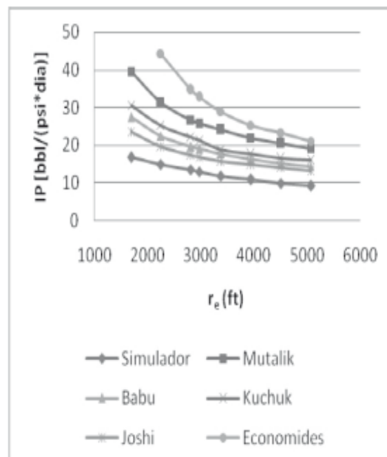
Figura 8. Comportamiento de la productividad del pozo variando el radio externo de frontera.
