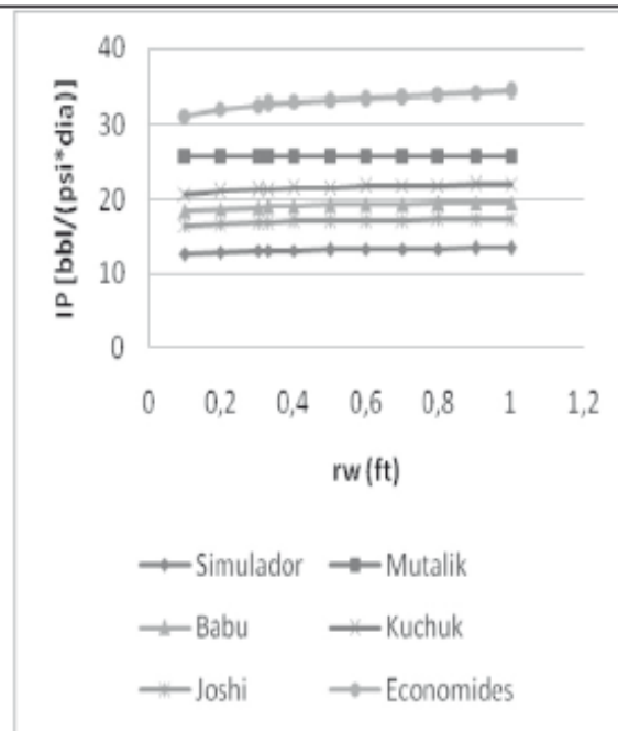
Figura 7. Comportamiento de la productividad del pozo variando el radio del pozo.
