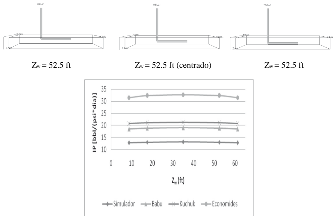
Figura 10. Comportamiento de la productividad del pozo variando la excentricidad en el eje vertical.
