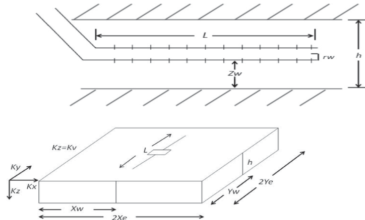
Figura 2. Esquema de un pozo horizontal localizado en un volumen rectangular de drenaje.
