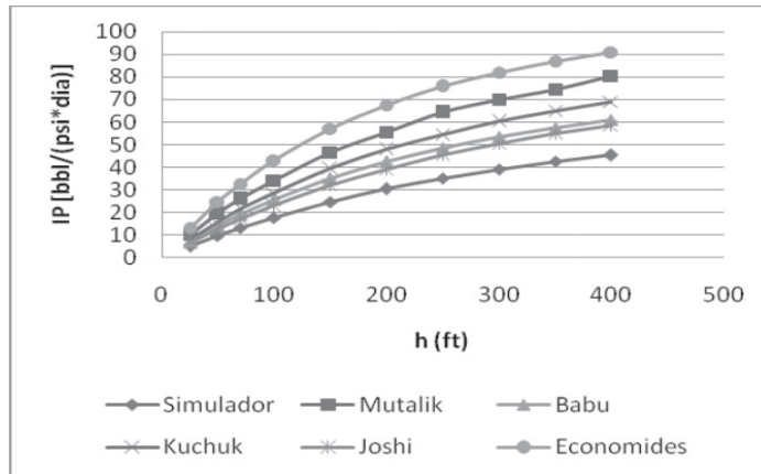
Figura 9. Comportamiento de la productividad del pozo variando el espesor de la capa.
